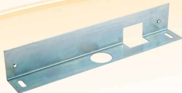
支架 尺寸：210x30x35(mm)
