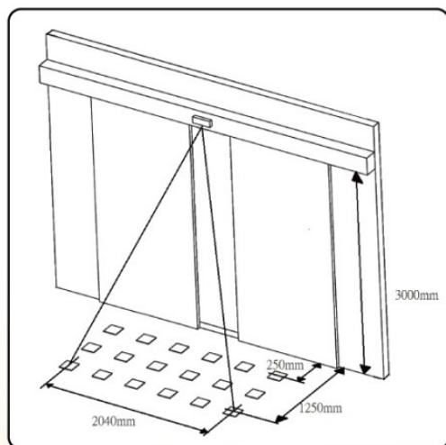
自動門視圖
